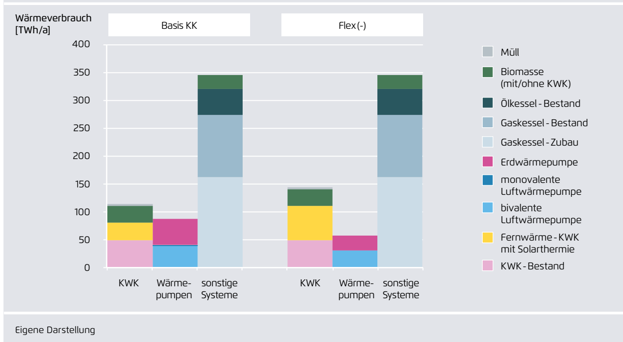
Zusammensetzung der Wärmeerzeugung in Haushalten und GHD-Gebäuden (Gewerbe, Handel, Dienstleitungen) in der Defizitvariante mit weniger dezentraler Flexibilität im Vergleich zum Basisszenario
