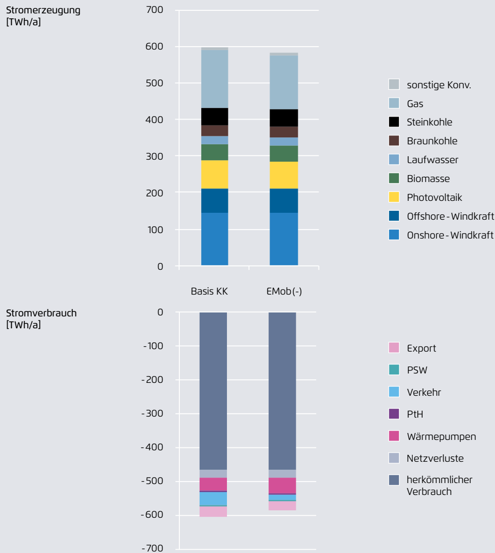
Erzeugte (oben) und verbrauchte (unten) Energiemengen in der Defizitvariante mit weniger E-Mobilität im Vergleich zum Basisszenario
