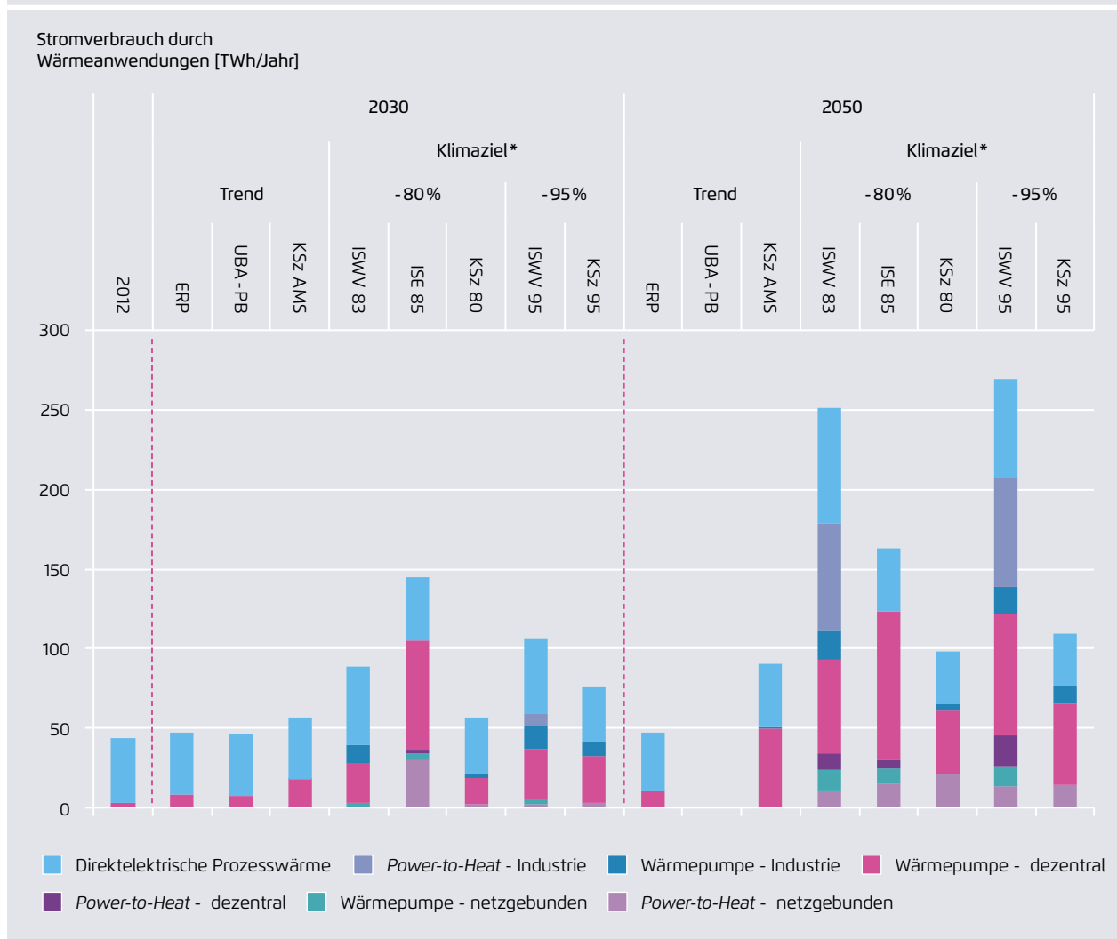
Szenarienvergleich: Stromverbrauch durch Wärmeanwendungen in Terawattstunden pro Jahr Abbildung 25
