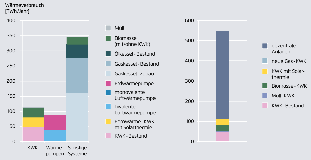
Zusammensetzung der Wärmeerzeugung in Haushalten und GHD-Gebäuden (Gewerbe, Handel, Dienstleitungen) im Basisszenario (Basis KK)
