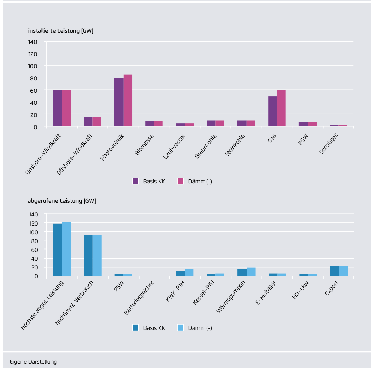
Installierte Erzeugungsleistungen (oben) und maximal abgerufene Verbrauchsleistungen (unten) für die Defizitvariante mit geringerer Dämmung im Vergleich zum Basisszenario
