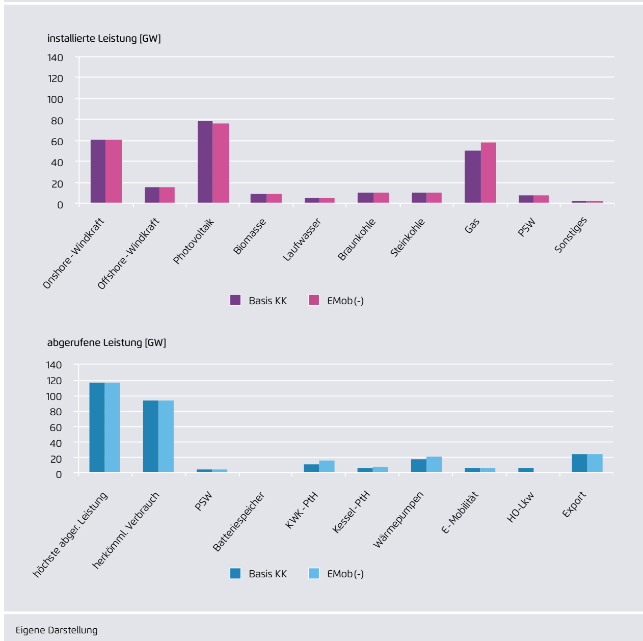
Installierte Erzeugungsleistungen (oben) und maximal abgerufene Verbrauchsleistungen (unten) für die Defizitvariante mit weniger E-Mobilität im Vergleich zum Basisszenario
